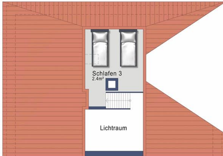
Dachgeschoss
